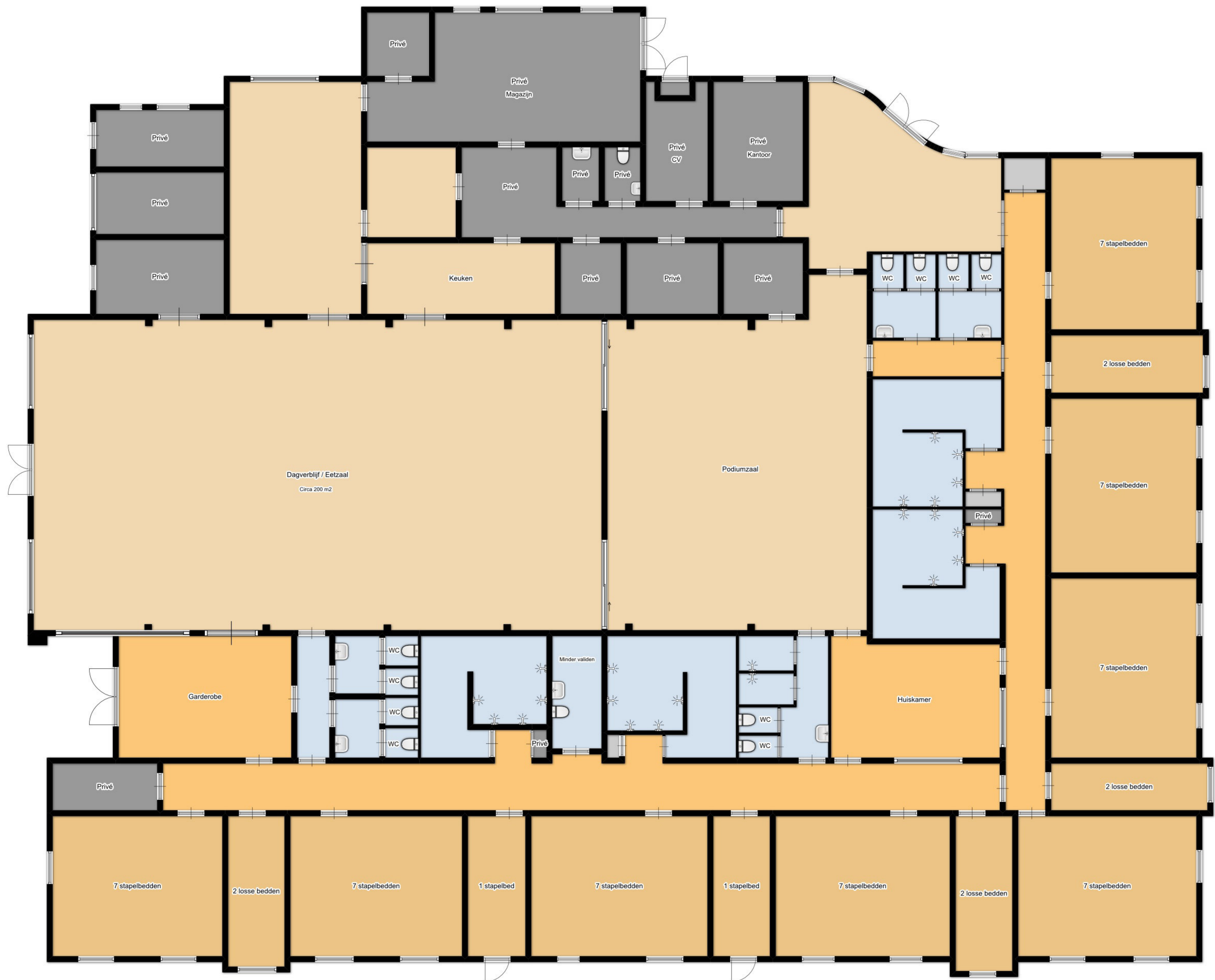
Plattegrond de Stulp
